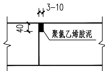
施工缝详图
