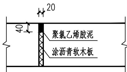
胀缝详图
