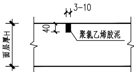
缩缝详图
