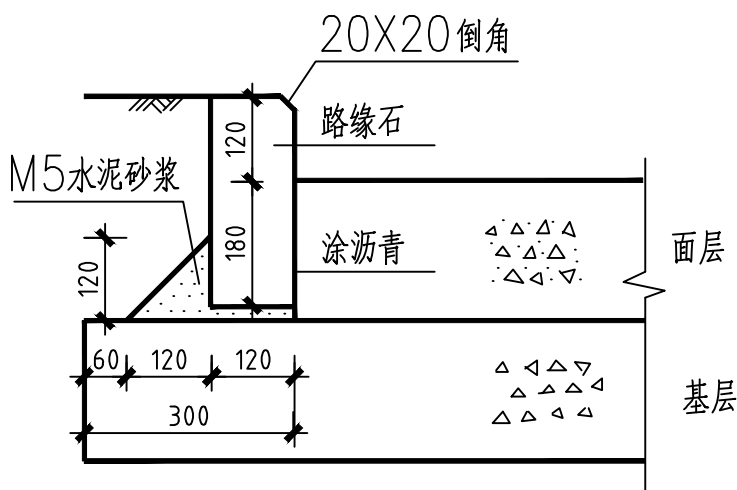
路缘石详图
