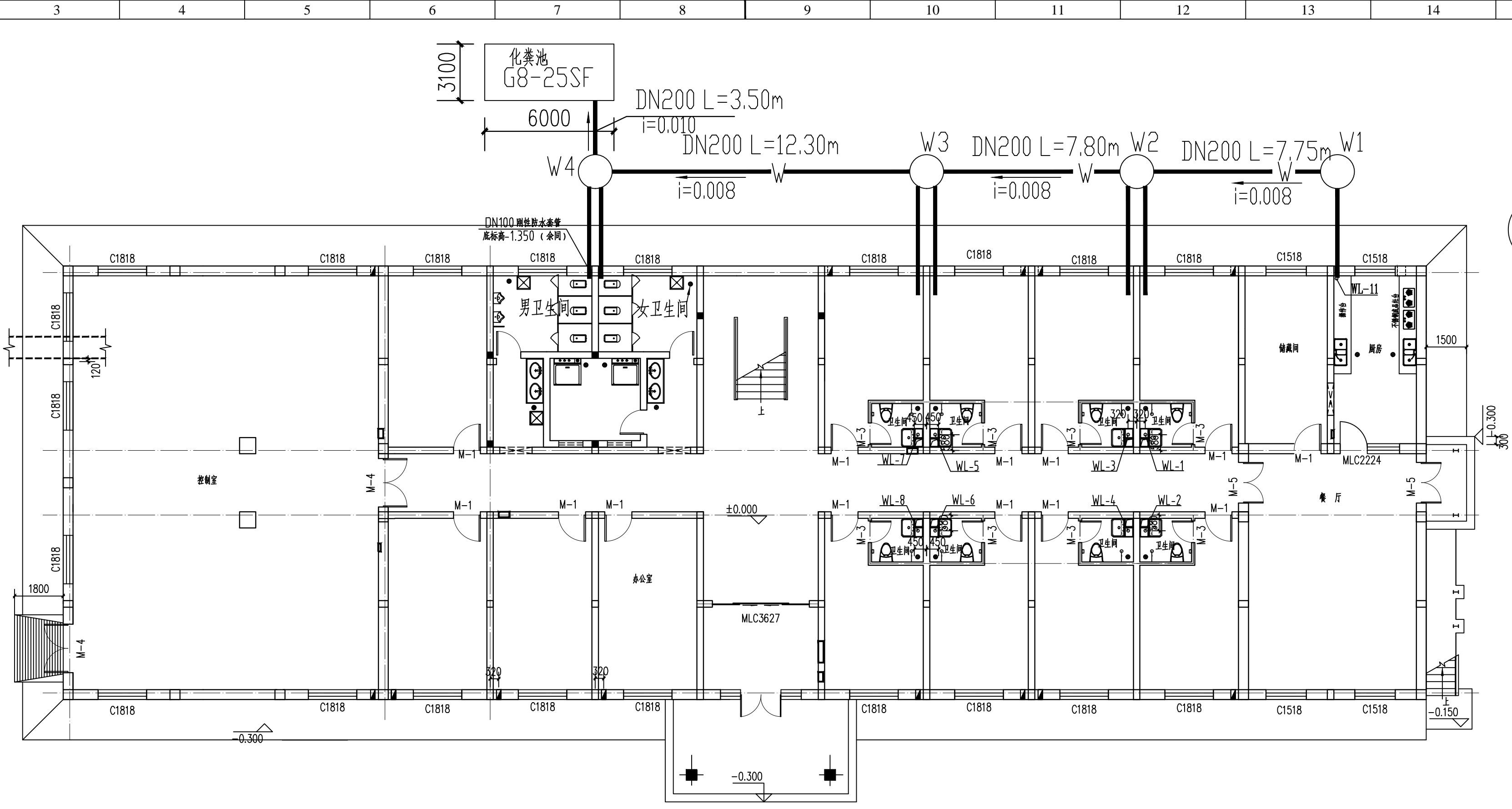
综合楼室外给排水平面图
