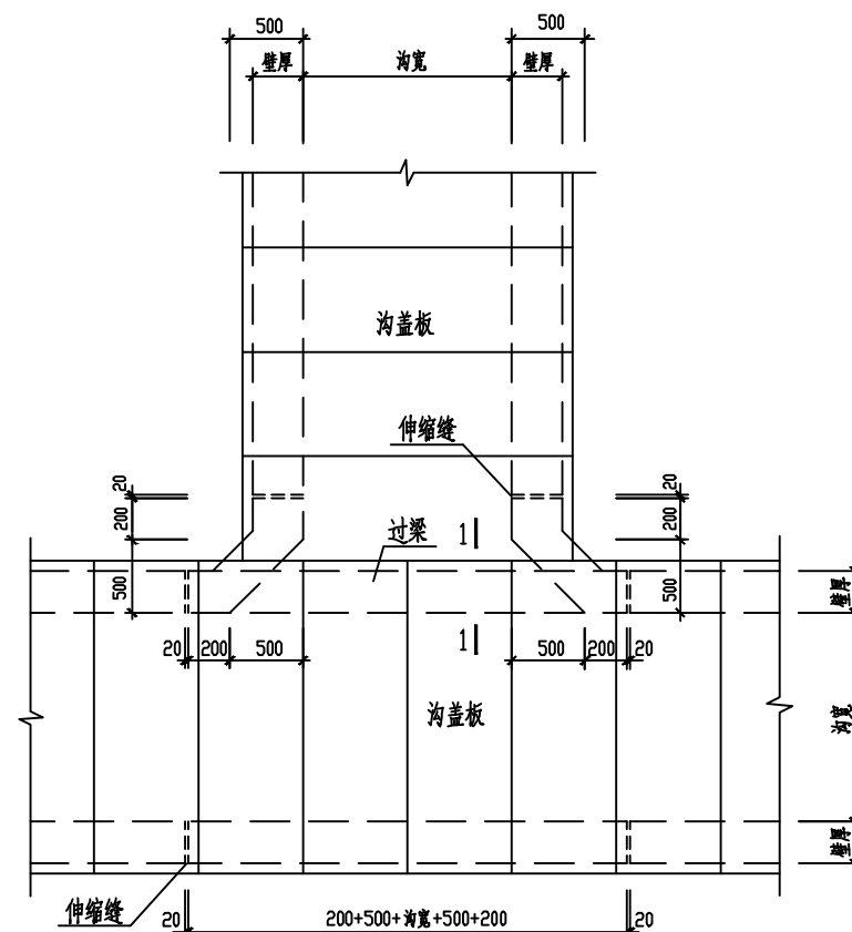
T形电缆沟交叉处处理详图 1:25
