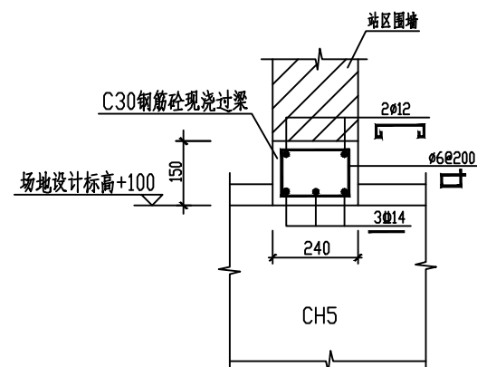
CH5电缆沟穿围墙处理图 1:10
