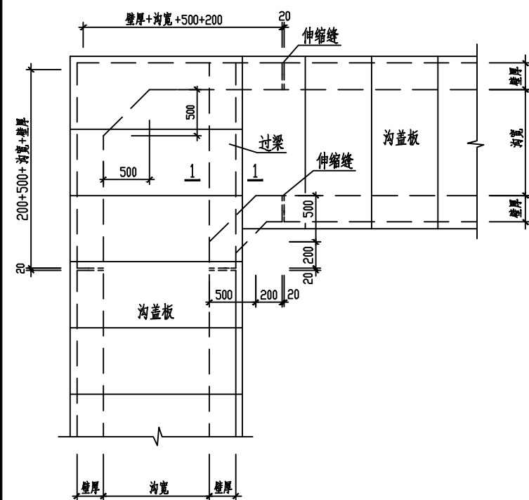
电缆沟直角交叉处处理详图 1:25
