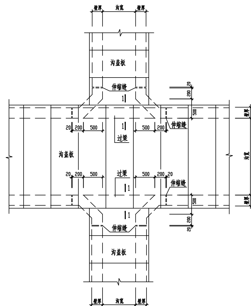
十字形电缆沟交叉处处理详图
