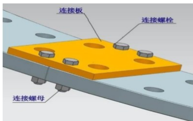
图 3.5 下锚板的拼接节点
