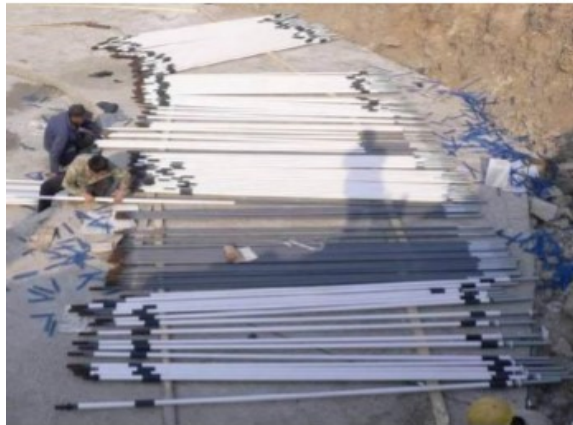
图 3.16 锚栓的准备工作图
