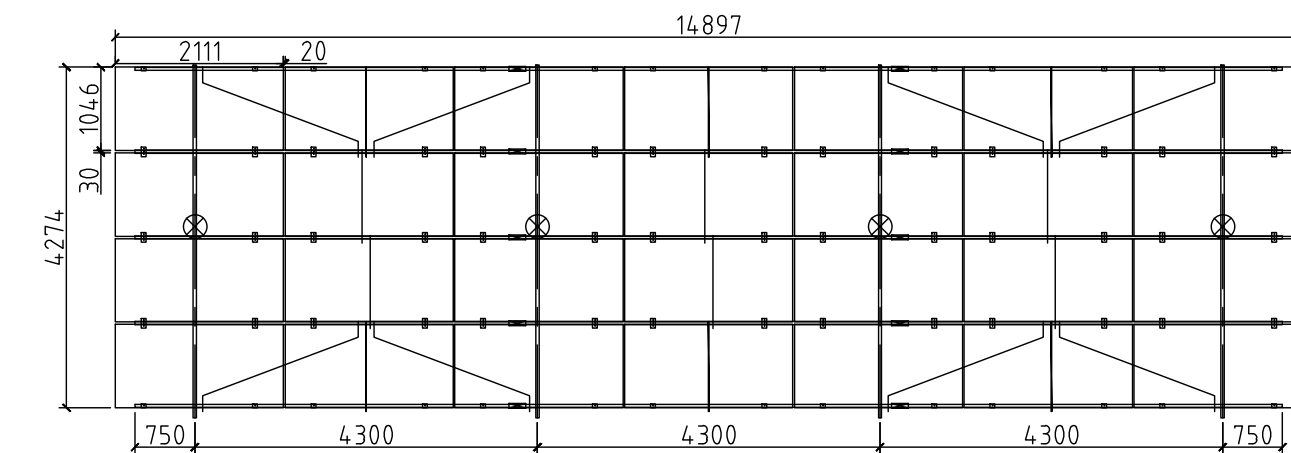
445Wp 组件4X7方阵桩基础布置图
