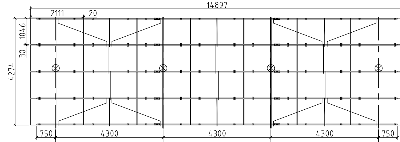
445Wp组件4X7方阵桩基布置图
