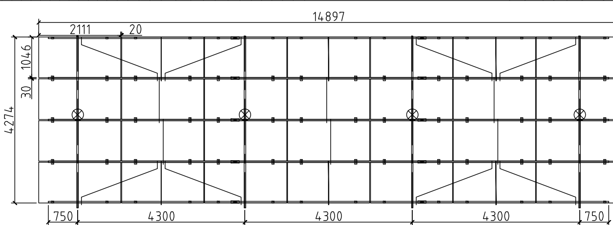
445Wp 组件4X7方阵桩基础布置图
