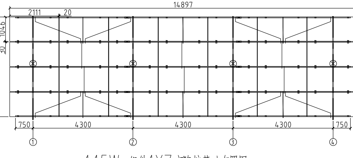
445Wp组件4X7方阵桩基础布置图
