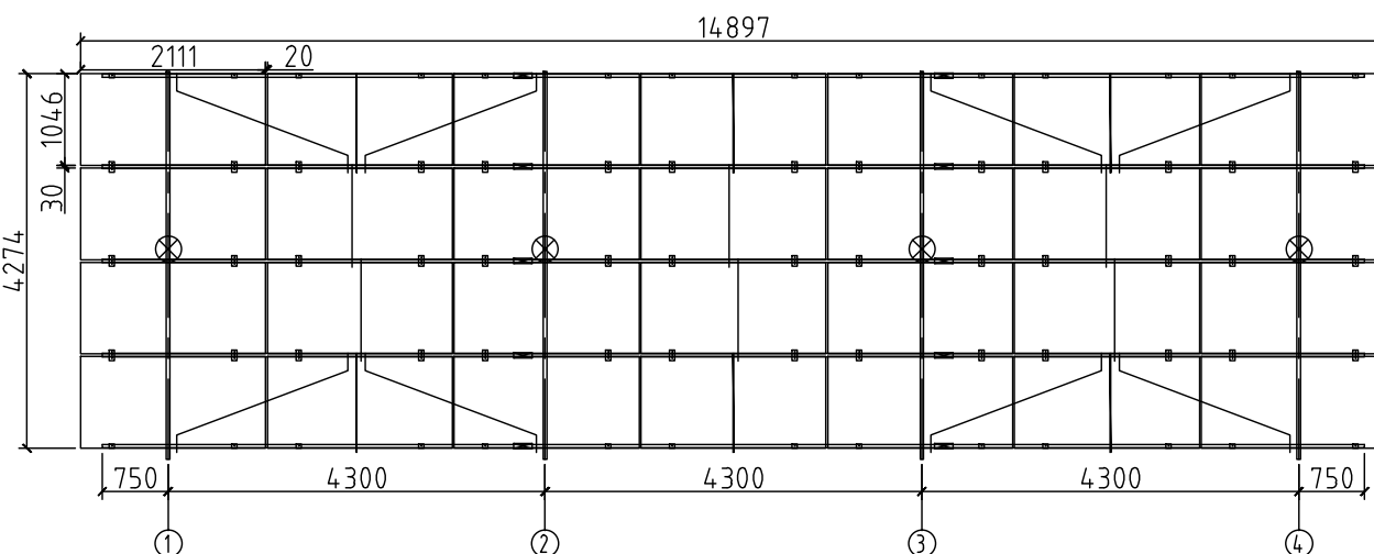
445Wp 组件4X7 方阵桩基础布置图
