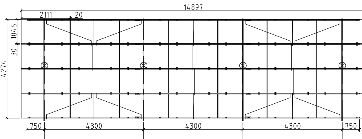
445W D 组件4×7方阵桩基础布置图
