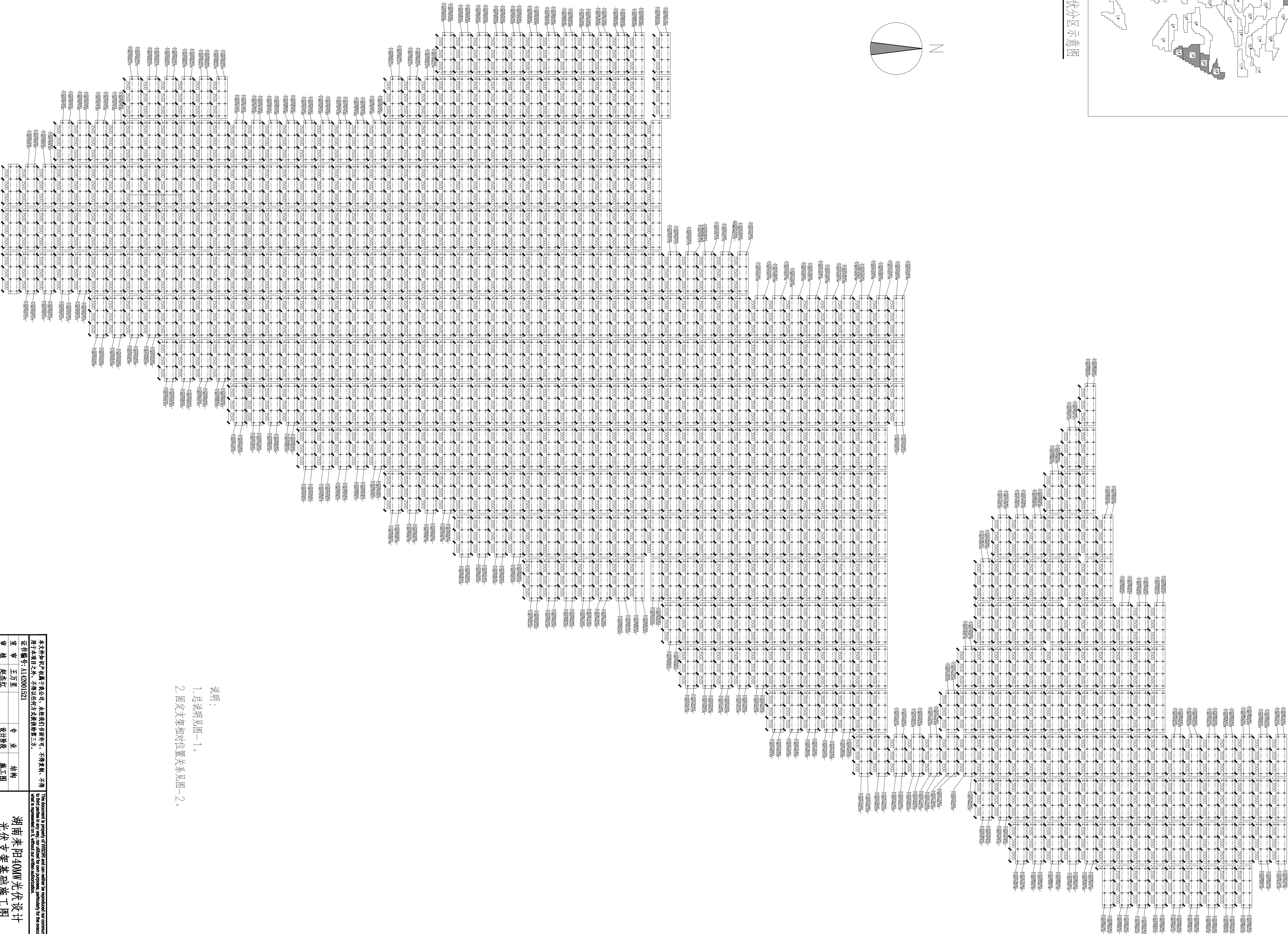
6#7#8#区域光伏支架平面布置图
