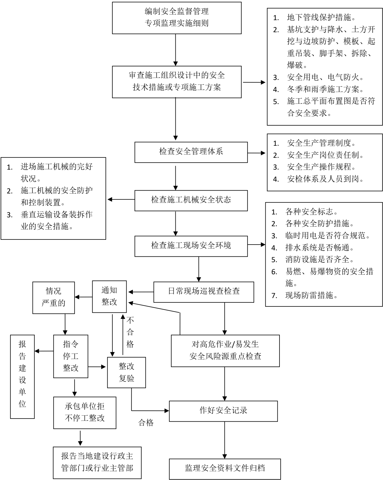
7-2 施工阶段工程安全监督管理程序框图
