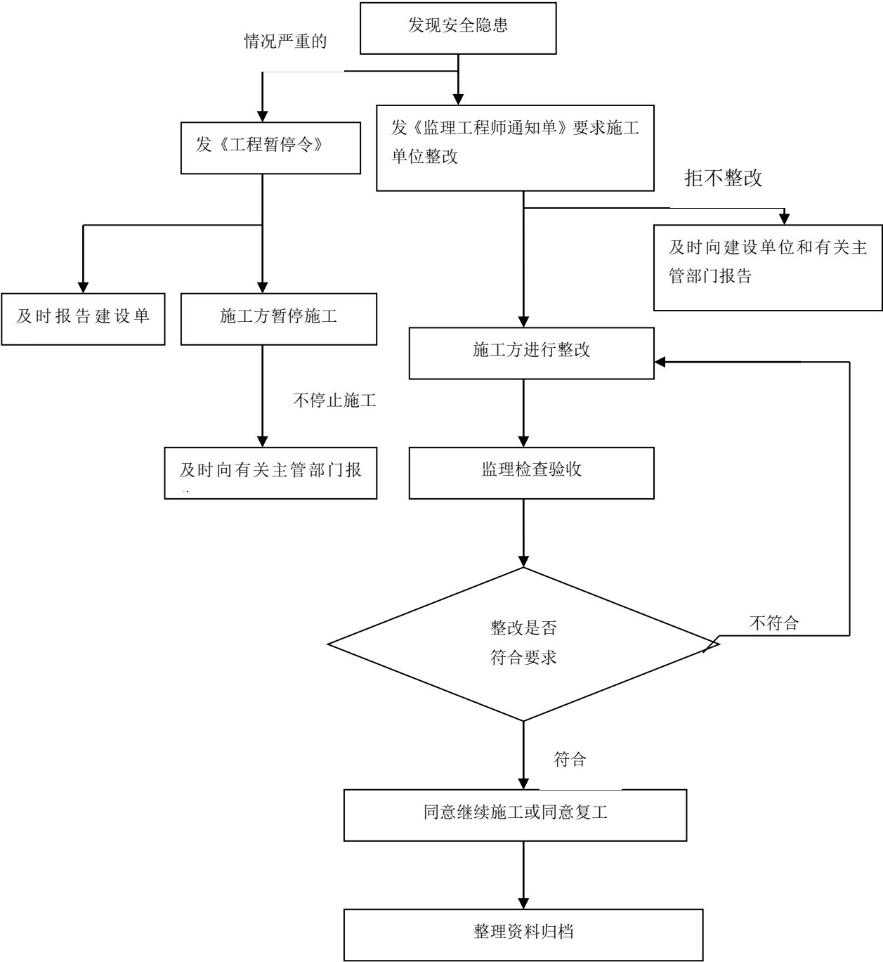
6-2 施工阶段工程安全监督管理程序框图
