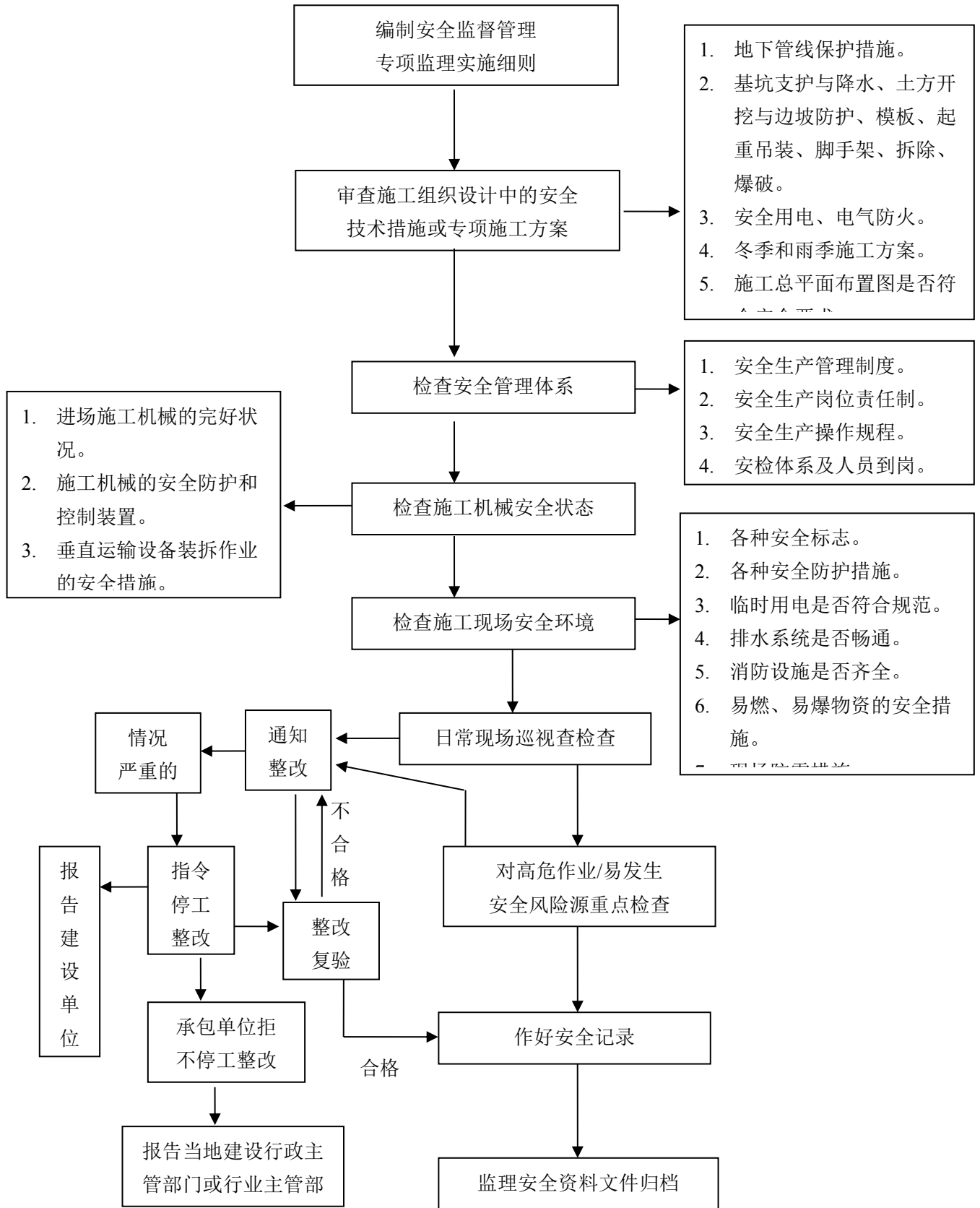
6-1 建设工程安全监督管理工作程序框图
