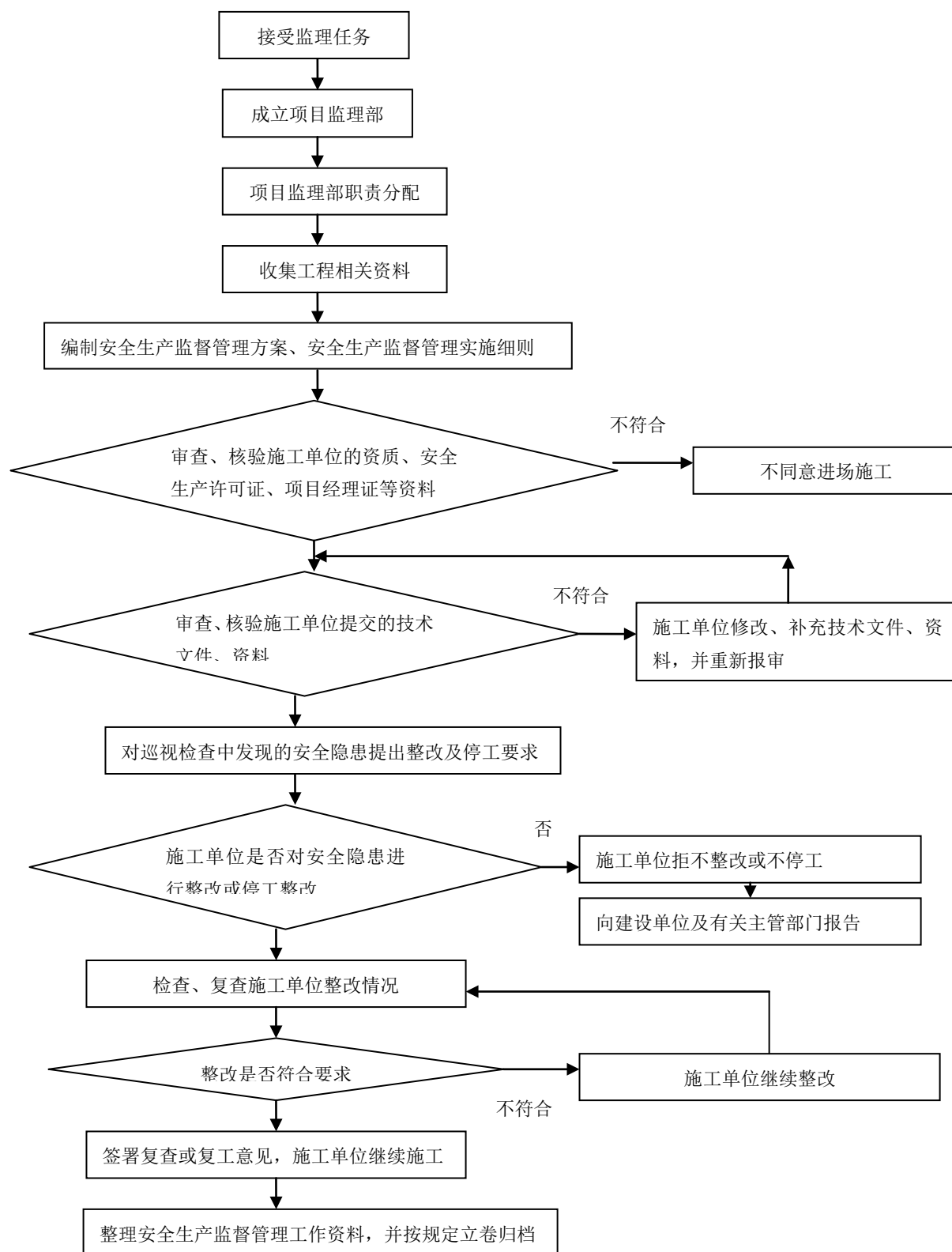
6.1 建设工程安全监督管理工作程序框图
