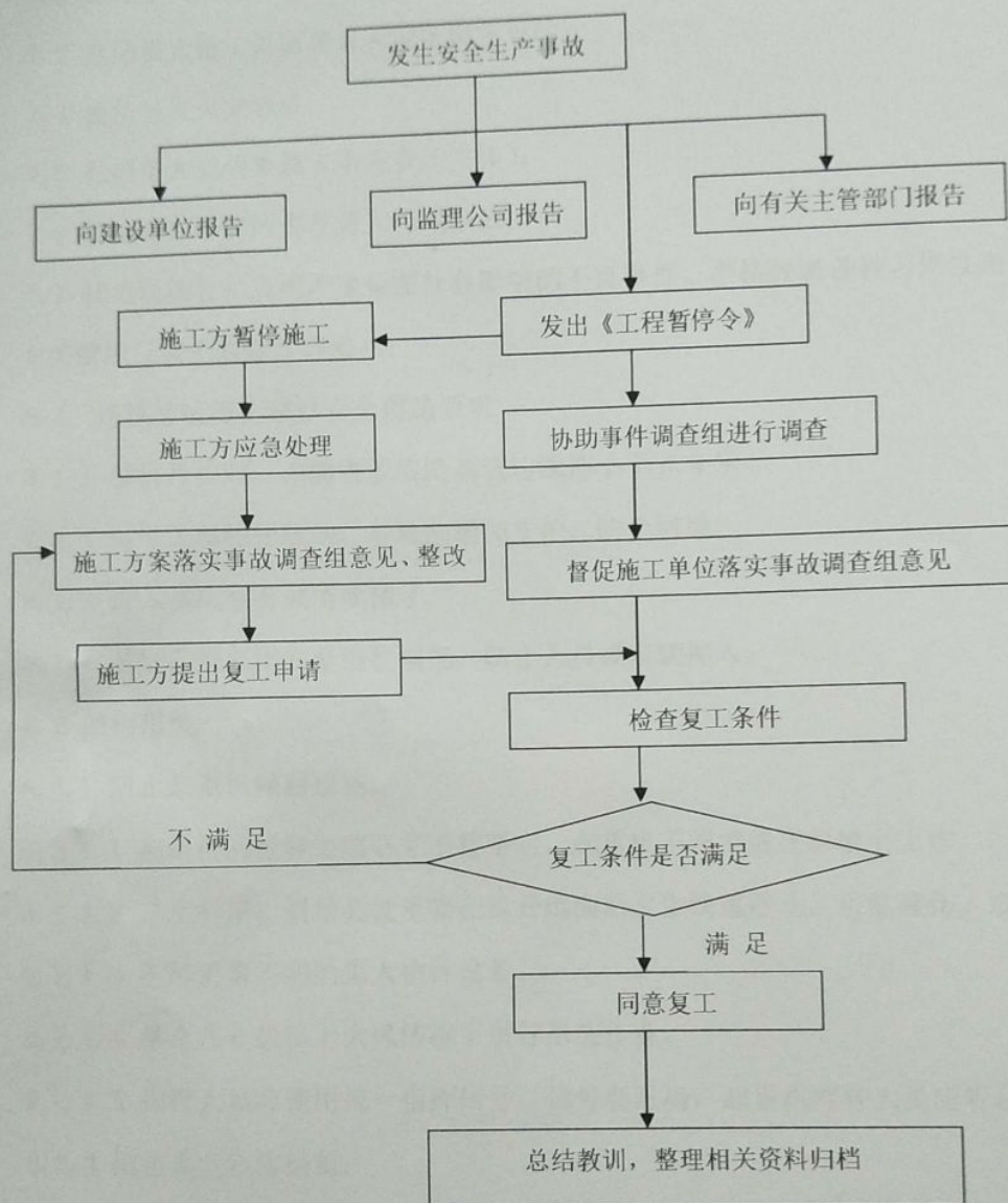
6-3 安全隐患处理程序图
