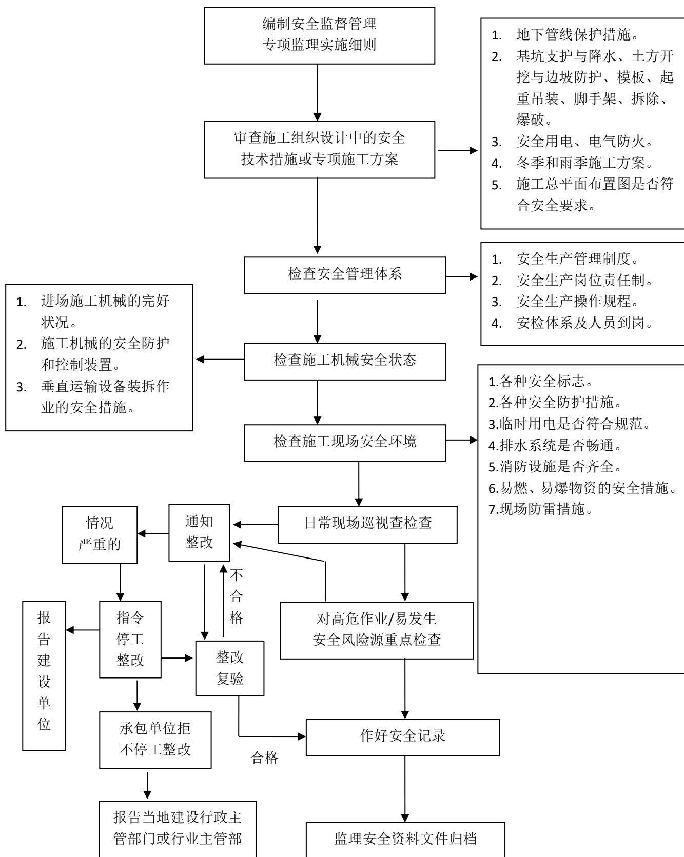
图 B.2 施工阶段工程安全监督管理程序框图
