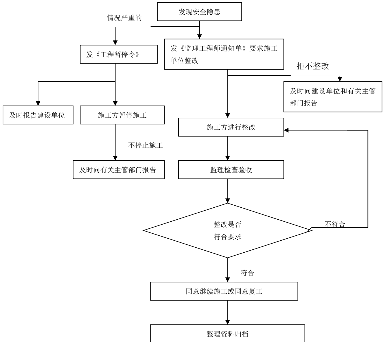
6-2 施工阶段工程安全监督管理程序框图
