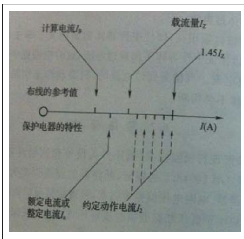
图 7 过电荷保护电器的动力特性关系图
