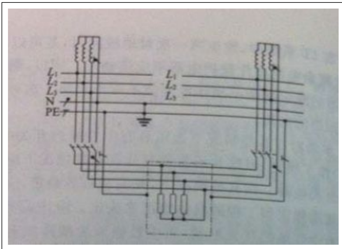
图2 在 TN-S 系统中，采用具有断开中性极的开关可避免产生杂散电流
