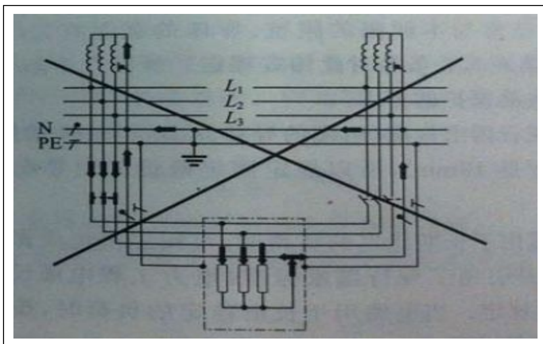
图 1 在 TN-S 系统中，产生杂散电流的例子
