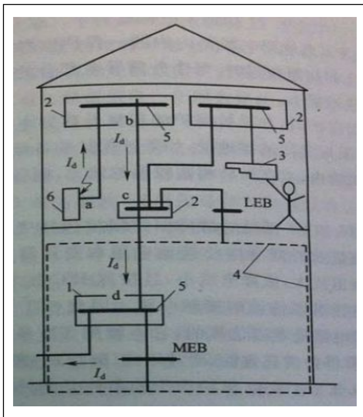
图 6 同一配电箱或配电干线间接引出的不同回路
