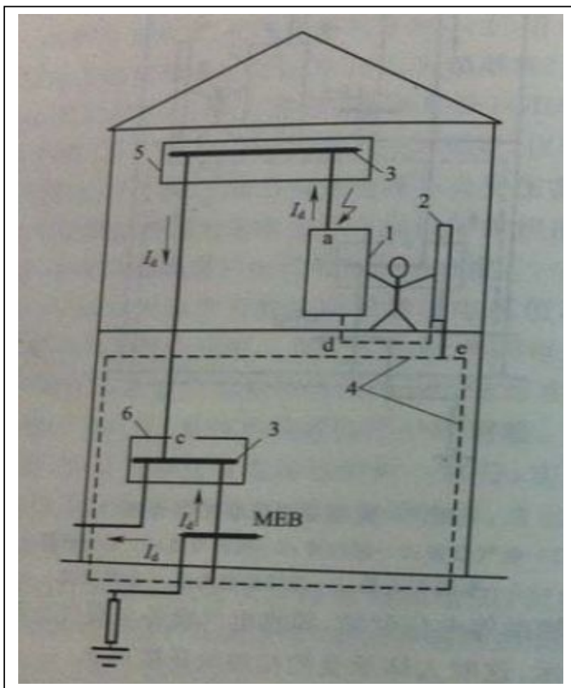
图4 辅助等电位联结的作用
