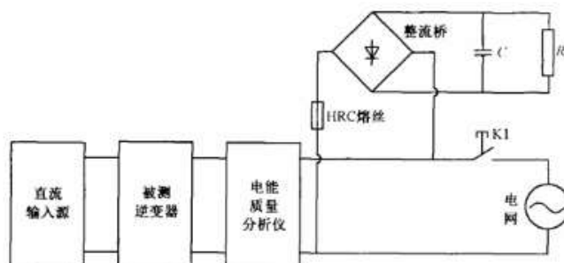
图4 暂态电压保护试验平台
