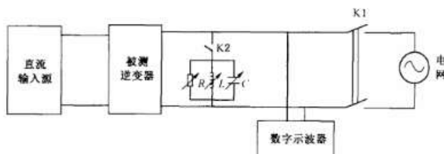
图3 防孤岛效应保护试验平台
