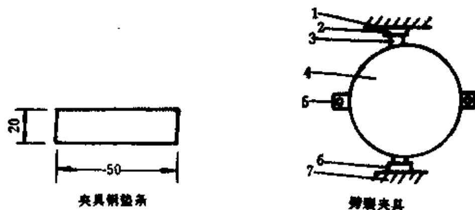
附图 6.2 混凝土劈裂抗拉试验装置示意图
