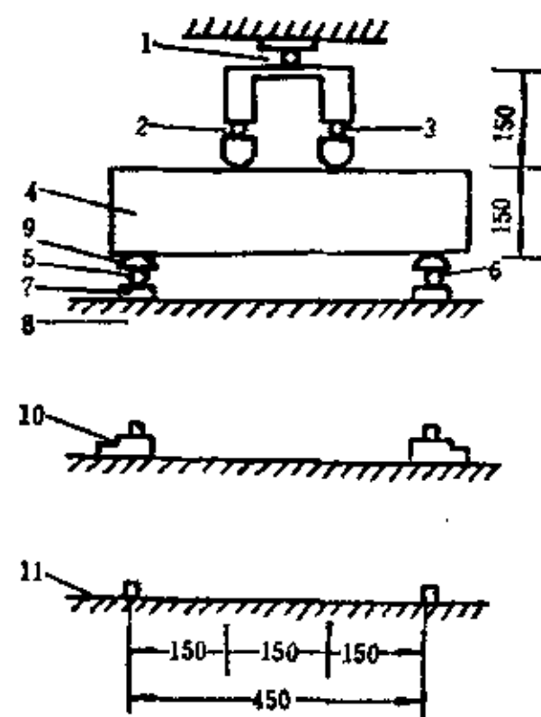
附图 6.1 抗折试验装置图(尺寸单位: mm)
