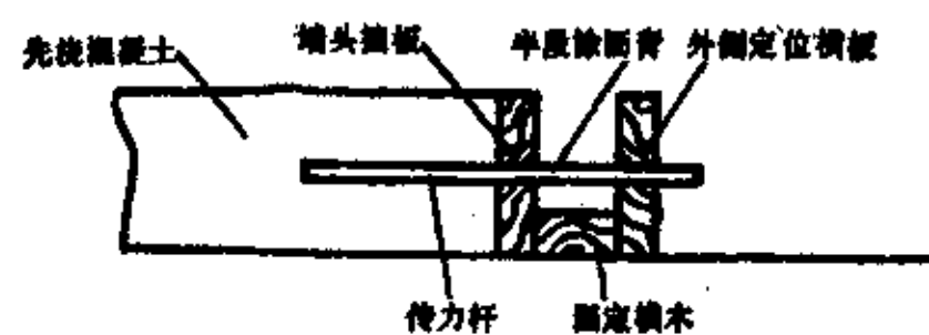
图 4.6.1-1 顶头木模固定传力杆安装图
