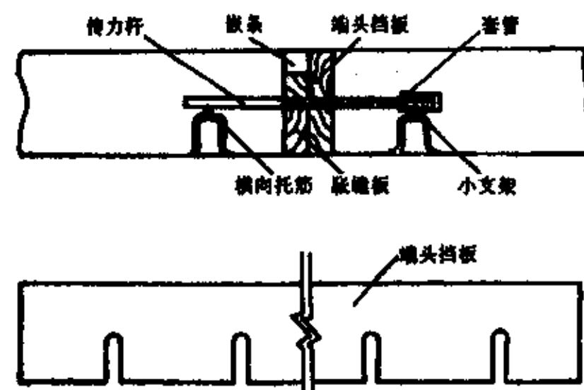
图 4.6.1-2 支架固定传力杆安装图
