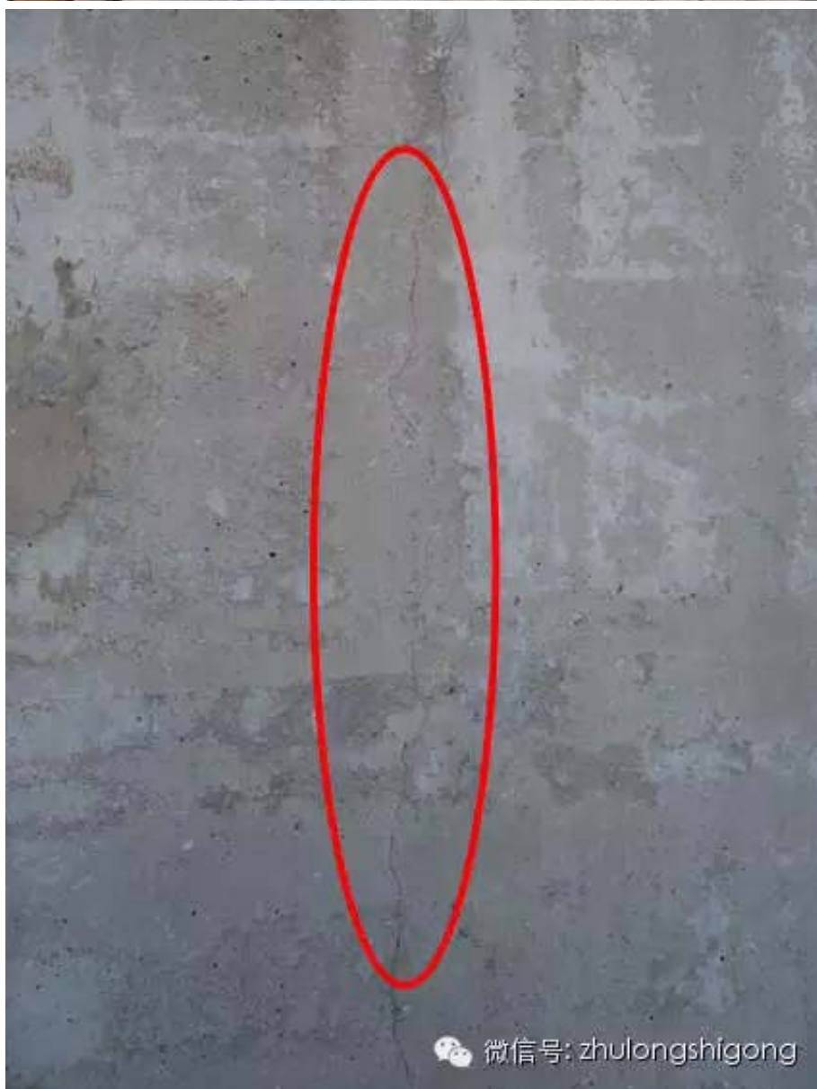
(7) 连接部位缺陷1：连接处混凝土缺陷，即烂根、错台等。
